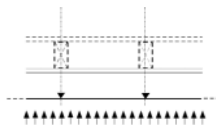
Abb 3.7.1: Beanspruchung als Platte
