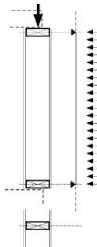
Abb. 3.7.2: Beanspruchung als Biegeträger mit Normalkraft
