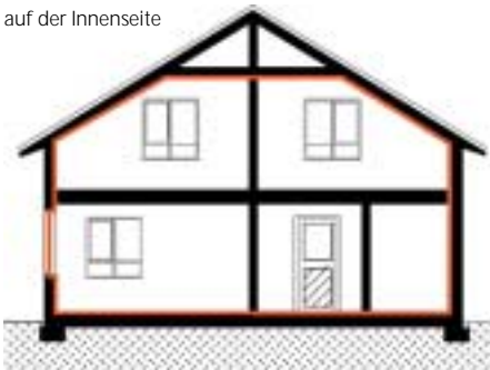
Abb. 3.1.6: Möglicher Verlauf der Luftdichtheitsebene in der Gebäudehülle.
