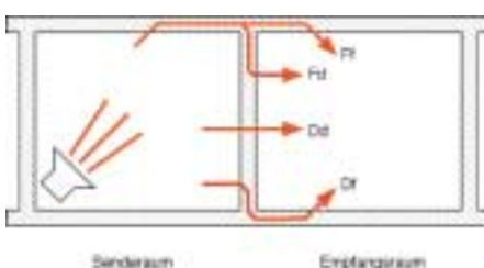
Abb. 3.5.1: Schallübertragungswege [47].
