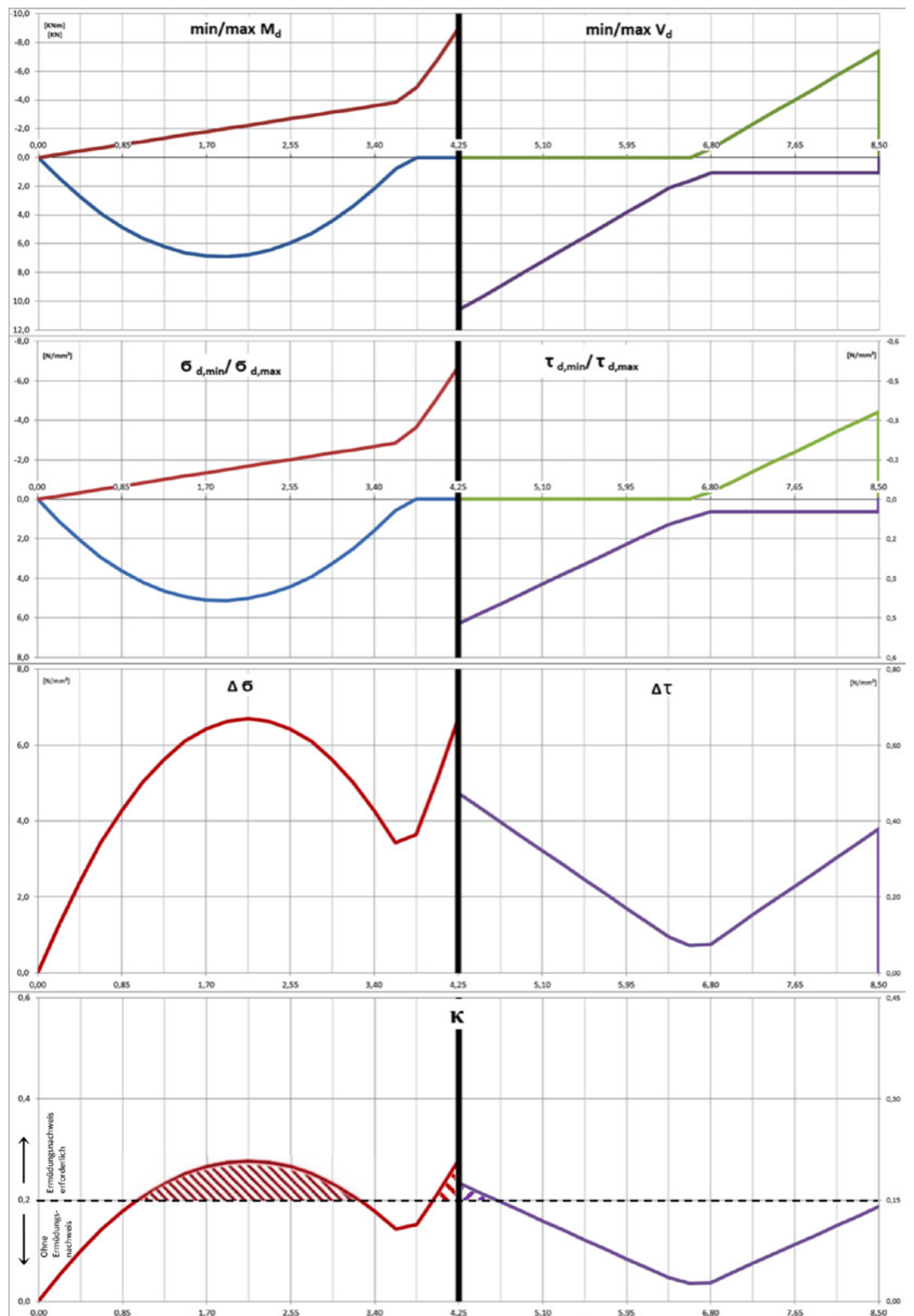
Bild 6.2: Schrittweise Durchführung des Ermüdungsnachweises beim 2-Feld-Träger
