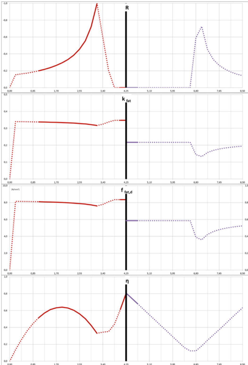
Bild 6.3: Schrittweise Durchführung des Ermüdungsnachweises beim 2-Feld-Träger
